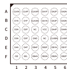
FO-36L
