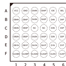
FO-36L
